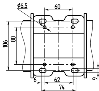
Рисунок 3. Вибратор ИВ-01-50Е.
